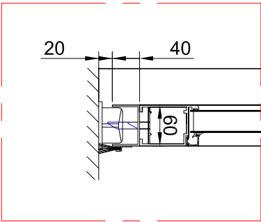
Boden ­ f hrung FOK fertig
