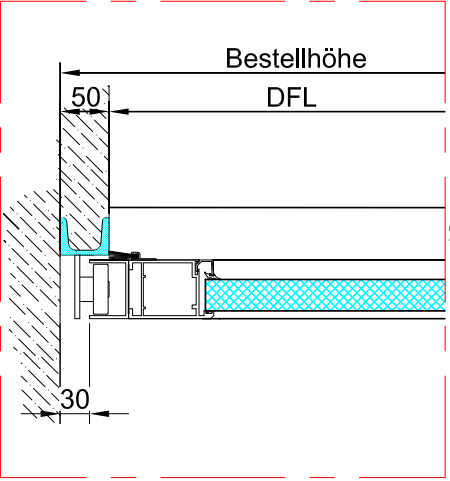
Schwelle Anschlagprofil U50
