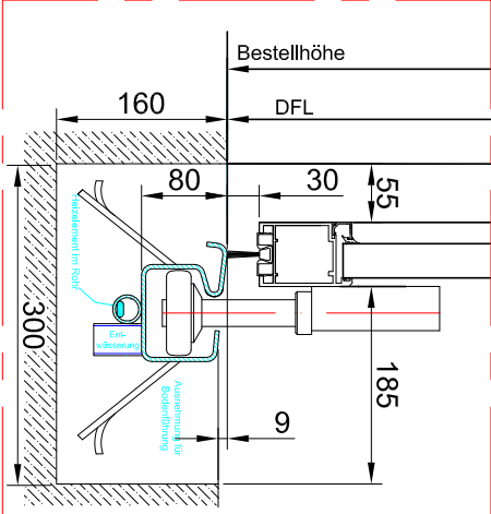
Boden ­ f hrung beheizt BF bhz
