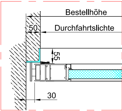
Schwelle Anschlagwinkel L50
