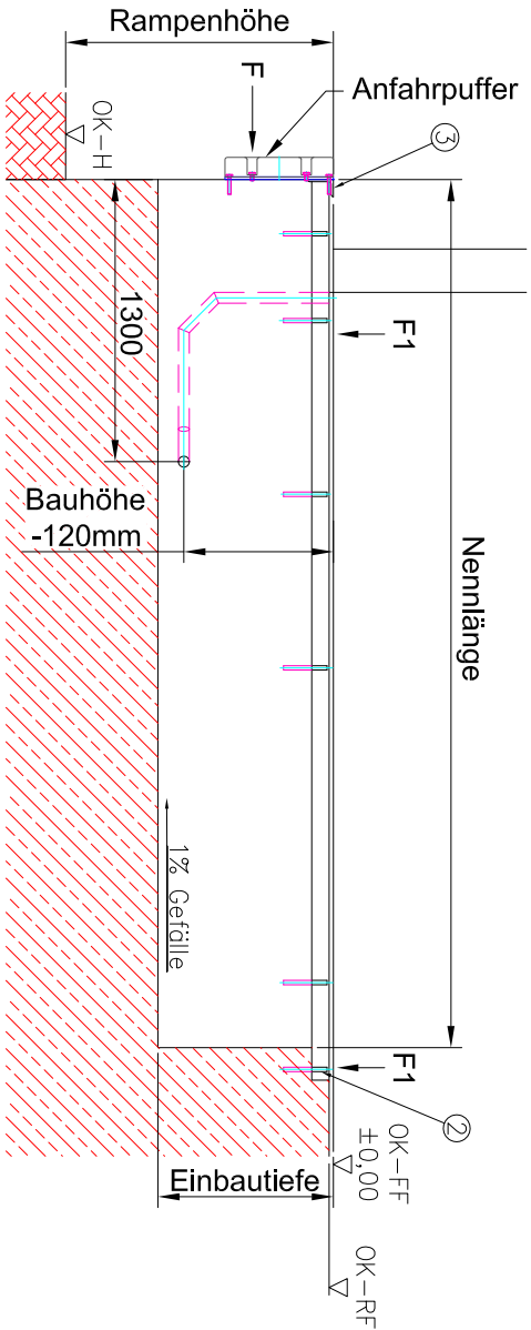
Schnitt A - A
