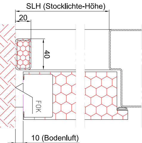
Aufbauschwelle Formrohr (20 mm) - Auswahl 2 Min. Bodeneinstand: ohne
