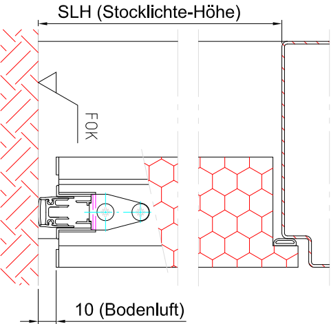
Absenkbare Bodendichtung Planet PU Beispiel Zarge mit Dichtnut, mit Bodentrennschiene
