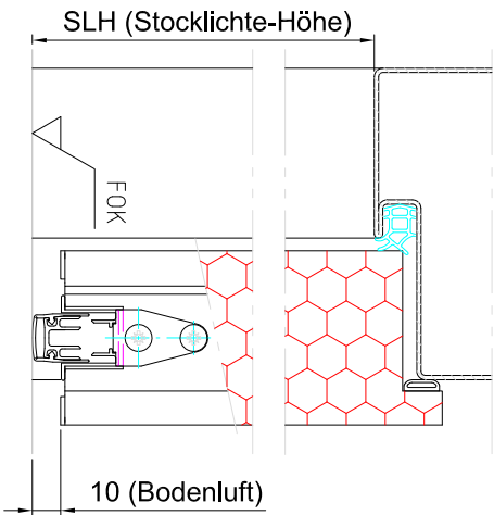
Absenkbare Bodendichtung Planet PU Beispiel Zarge mit Dichtnut, mit Bodentrennschiene
