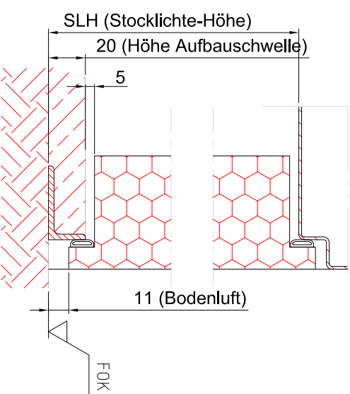
Aufbauschw. Winkel (20)+TB vierseitig-Ausw. 11 Min. Bodeneinstand: ohne
