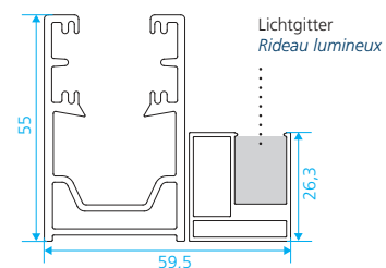
Rideau lumineux avec coulisseeux 34 x 55 mm
