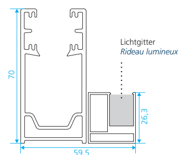
Rideau lumineux avec coulisseeux 34 x 70 mm
