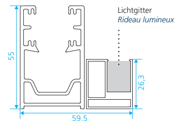
Rideau lumineux avec coulisseaux 34 x 55 mm
