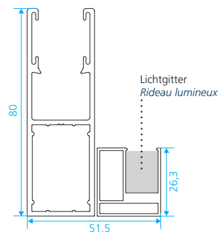
Rideau lumineux avec coulisseaux 26 x 80 mm
