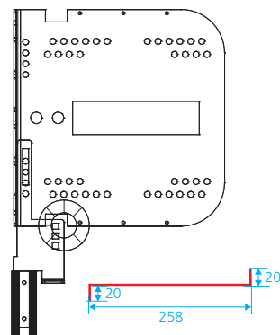
Untersichtsblende
