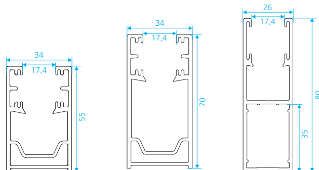
Standard-Führungsschiene
