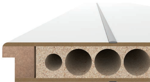
Schnitt Metaopt, Standardeinlage RSP
