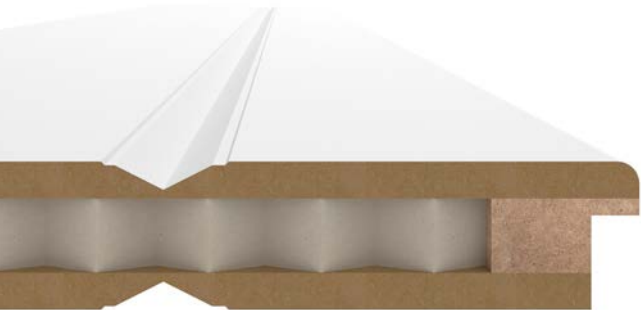
Schnitt Country, Standardeinlage Wabe
