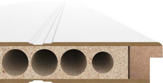
Schnitt Chello, Standardeinlage RSP
