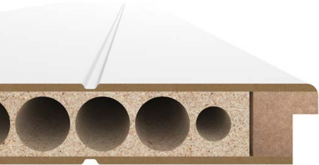
Schnitt Luana, Standardeinlage RSP
