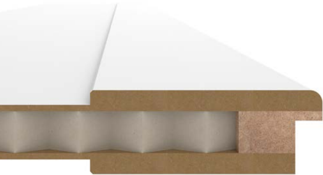
Schnitt Classic, Standardeinlage Wabe
