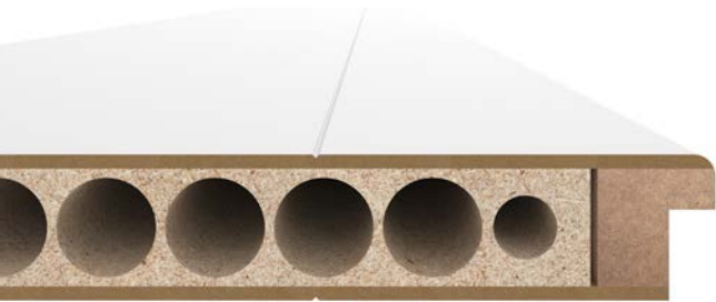
Schnitt Gap, Standardeinlage RSP
