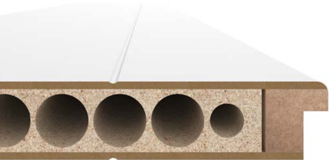
Schnitt Linje, Standardeinlage RSP
