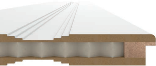
Schnitt Finesse, Standardeinlage Wabe
