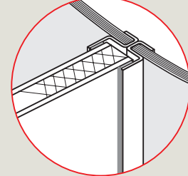
ohne Nachtabschluss
