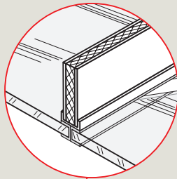
oberer Fassadenanschluss
