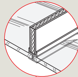
oberer Fassadenanschluss
