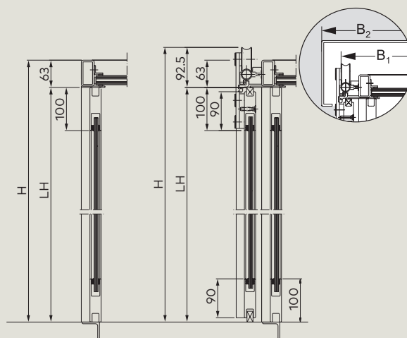
Seitenwand mit Sicherheitsglasfüllung
