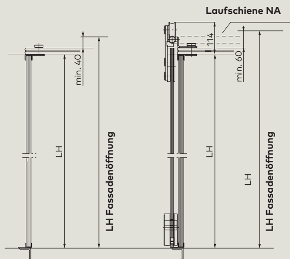
Seitenwand mit Sicherheitsglasfüllung
