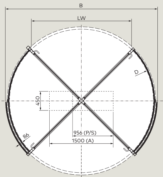
Seitenwand mit Sicherheitsglasfüllung
