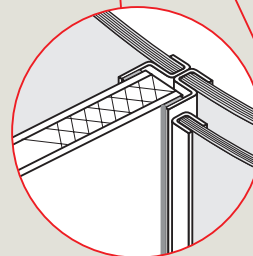
Nachtabschluss außen
