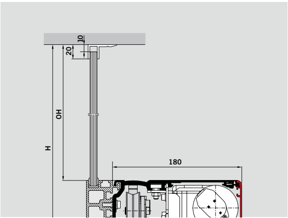
Avec imposte
