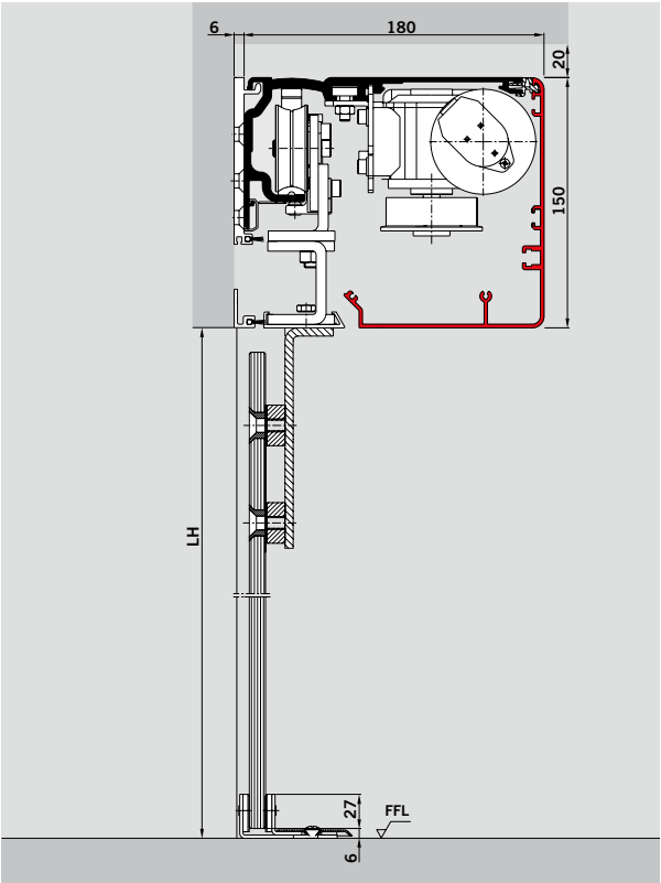
Montage en applique Opérateur 150 mm
