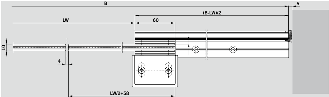
Coupe horizontale avec partie fixe
