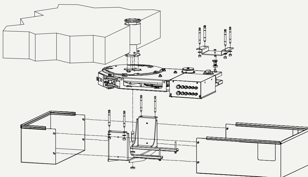
Antrieb unterflur
