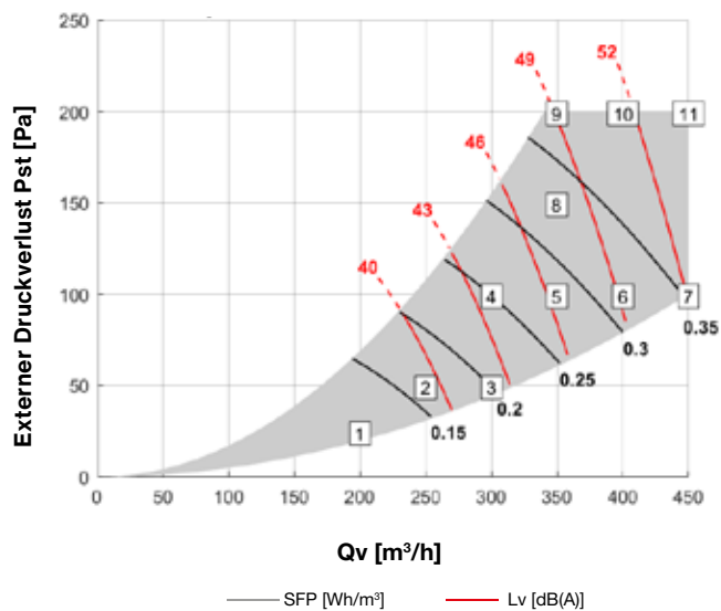
Leistungsdiagramm ComfoClima 36 mit ComfoAir Q 450
