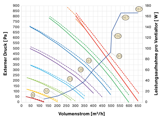
Zehnder ComfoAir Q 600 mit Zehnder ComfoClima 36
