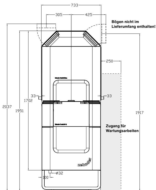
Frontansicht Zehnder ComfoClima 36
