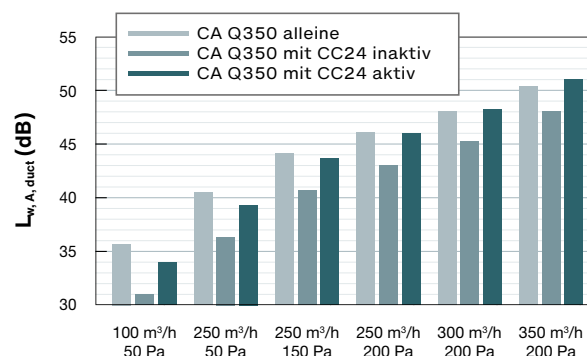
Geräuschpegel Abluft Zehnder ComfoAir Q350 mit und ohne Zehnder ComfoClima 24
