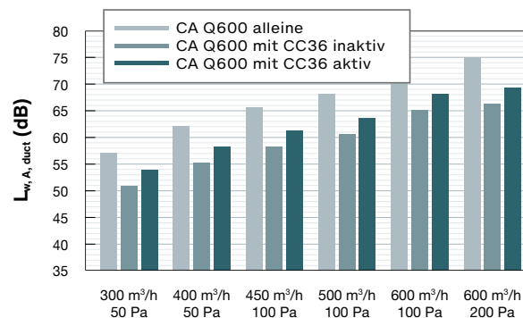
Geräuschpegel Zuluft Zehnder ComfoAir Q 600 mit und ohne Zehnder ComfoClima 36
