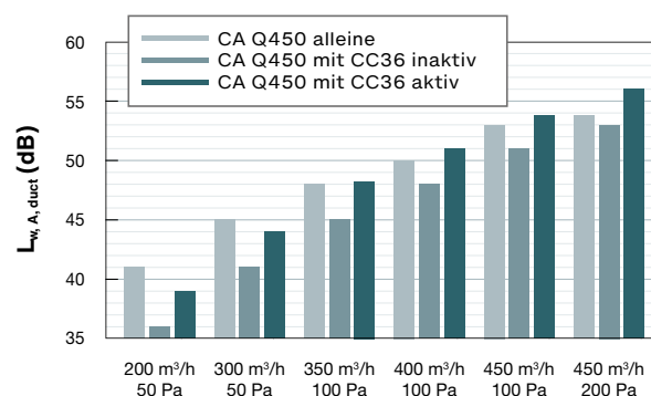
Geräuschpegel Abluft Zehnder ComfoAir Q450 mit und ohne Zehnder ComfoClima 36
