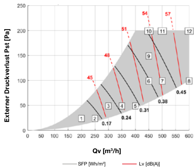
Leistungsdiagramm ComfoClima 36 mit ComfoAir Q 600
