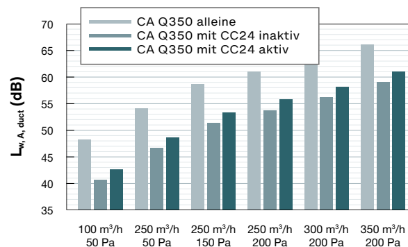
Geräuschpegel Zuluft Zehnder ComfoAir Q350 mit und ohne Zehnder ComfoClima 24
