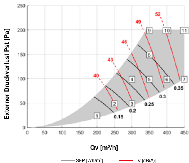
Leistungsdiagramm ComfoClima 24 mit ComfoAir Q 450
