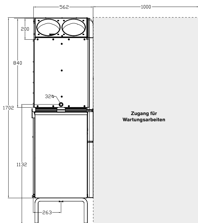
Seitenansicht
