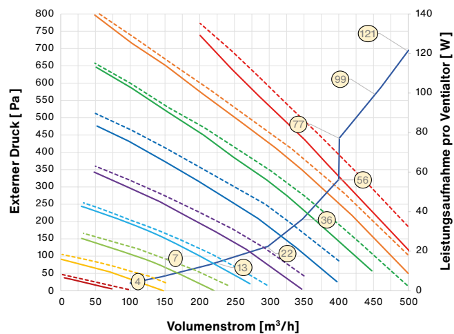
Zehnder ComfoAir Q 450 mit Zehnder ComfoClima 24
