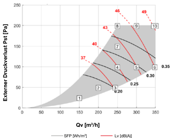
Leistungsdiagramm ComfoClima 24 mit ComfoAir Q 350
