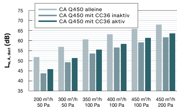
Geräuschpegel Zuluft Zehnder ComfoAir Q450 mit und ohne Zehnder ComfoClima 36
