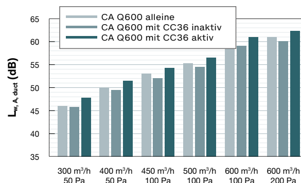
Geräteabstrahlung Zehnder ComfoAir Q 600 mit und ohne Zehnder ComfoClima 36
