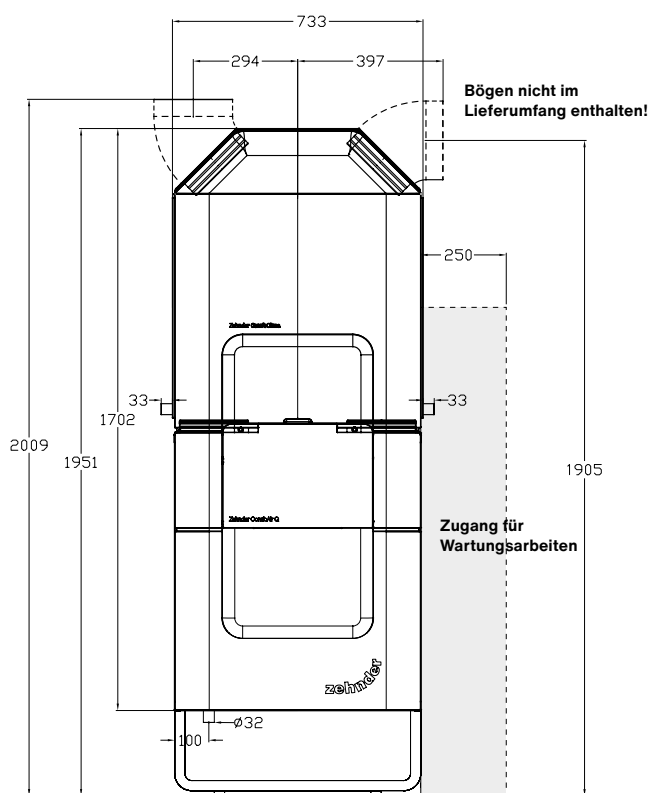
Frontansicht Zehnder ComfoClima 24
