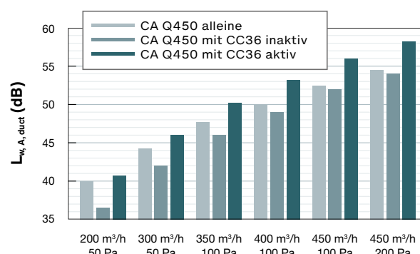
Geräteabstrahlung Zehnder ComfoAir Q450 mit und ohne Zehnder ComfoClima 36
