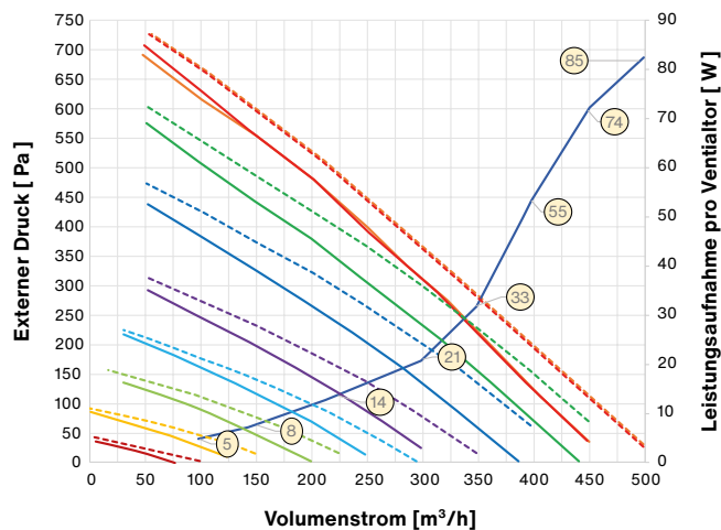
Zehnder ComfoAir Q 350 mit Zehnder ComfoClima 24
