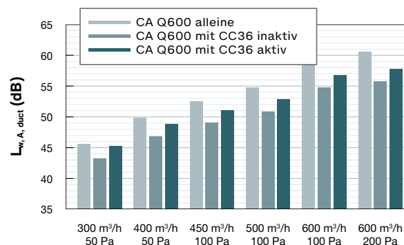
Geräuschpegel Abluft Zehnder ComfoAir Q 600 mit und ohne Zehnder ComfoClima 36
