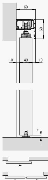
Hawa Porta 100 HC
