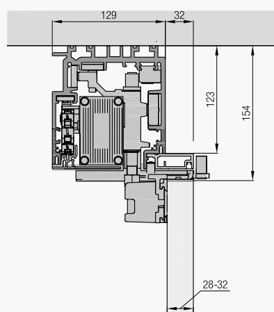
Hawa Frontego 30
