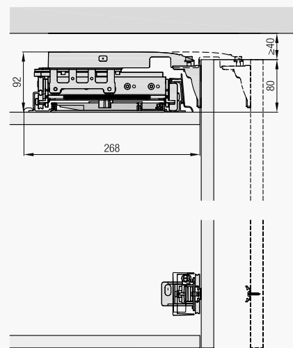
Hawa Frontino 20 H OS FS
