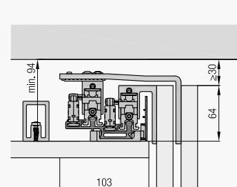
Hawa Combino 80 H FS ol
