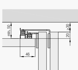
Hawa Combino 50 H FS avec amortissement
