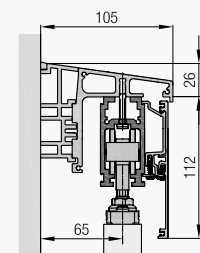
Hawa Frontslide 60 A/matic
