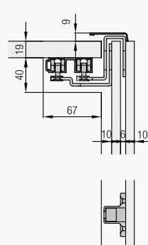
Hawa Clipo 16 H FS 2 voies
