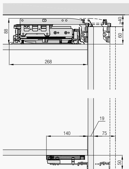
Hawa Frontino 20 H FS rh
