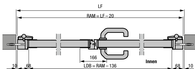
2-flügelige Nebentür mit Aluminium-Blockzarge Profiltyp 2 Einbau in der Öffnung
