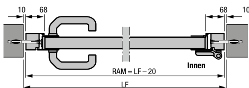
Nebentür mit Aluminium-Blockzarge Profiltyp 2 Einbau in der Öffnung
