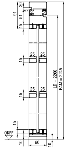
Vertikalschnitt 1-flügelige Stahl-Lofttür
