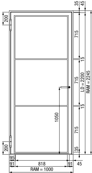
1-flügelige Stahl-Lofttür
