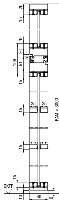
Vertikalschnitt 1-flügelige Stahl-Lofttür mit Seitenteilen und Oberlicht
