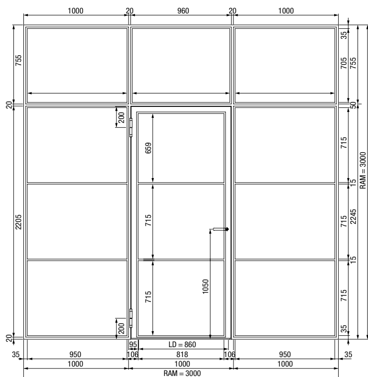
1-flügelige Stahl-Lofttür mit Seitenteilen und Oberlicht
