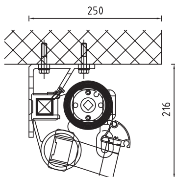
DECKENMONTAGE
