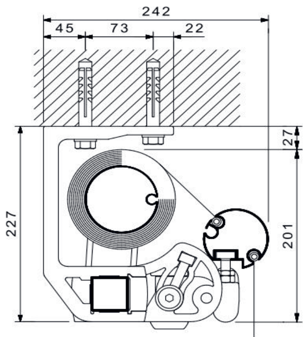
Deckenmontage
