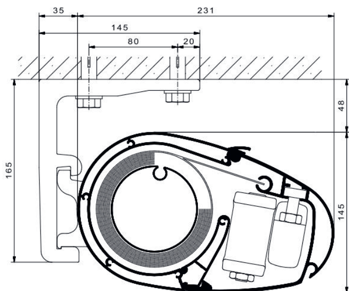
Deckenmontage
