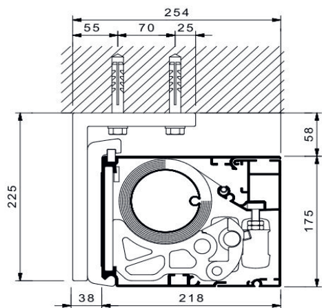
Deckenmontage
