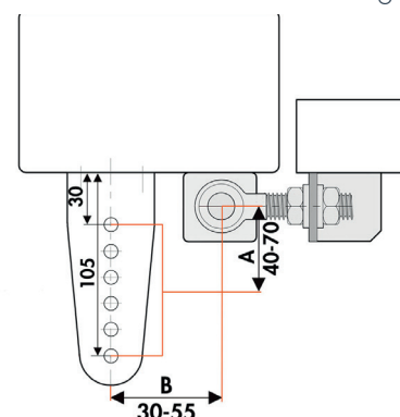
Bandposition 3: Anbau Türschließer DIREKT 150 an Zugangstüren mit Augenschraubenbändern
