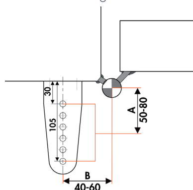
Bandposition 1: Anbau DIREKT 150 an Zugangstüren mit einseitigen Bändern
