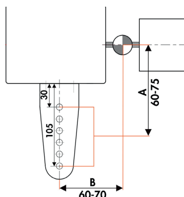
Bandposition 2: Anbau Türschließer DIREKT 150 an Zugangstüren mit mittig angebrachten Bändern
