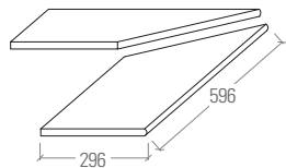
Angolo esterno bordo con toro 30x60
