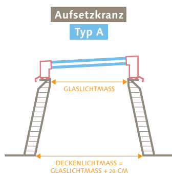
POLYESTERZARGE KONISCH * Höhen: 15/30/50 cm
