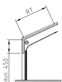
Normalbeschlag NB-DF mit Dachfolge
