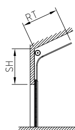
Hebungsbeschlag HB-DF mit Dachfolge
