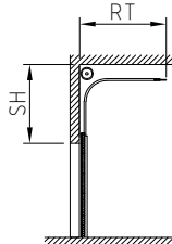
Hebungsbeschlag HB
