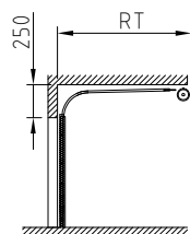
Niedrigbeschlag NSB
