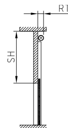
Vertikalbeschlag VL
