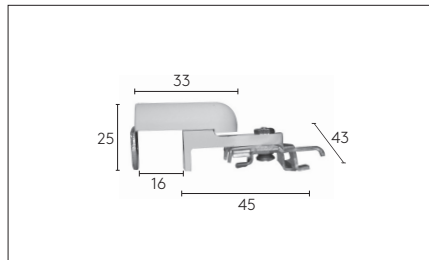
Klemm-Klebeträger oben Art.-Nr. 14.3247
