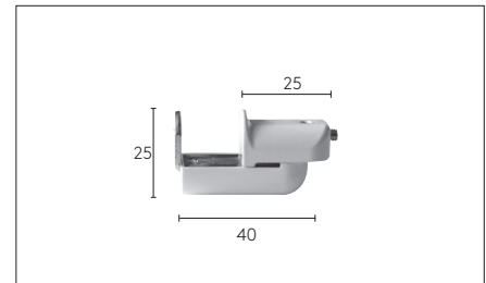
Klemm-Klebe-Abspannwinkel unten Art.-Nr. 15.0921
