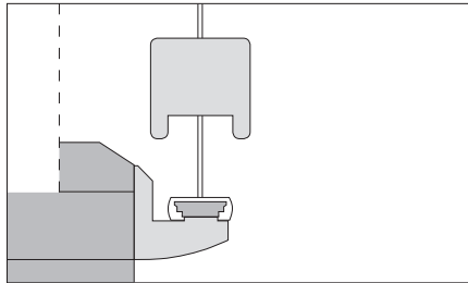
Schnitt Fensterrahmen mit Kunststoffträger und Unterschiene
