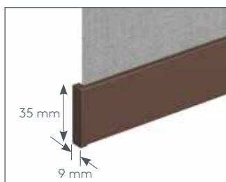
Unterleiste CUBUS-U
