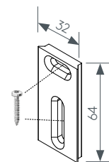
Abb. Montageplatte für Wandmontage
