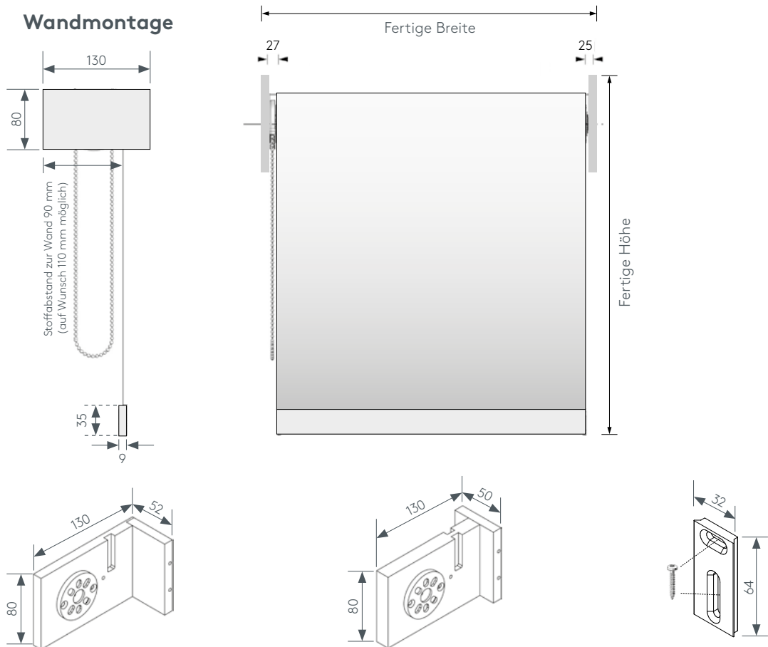
Abb. Wandträger
