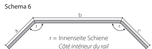
Vermassung: aussen und Sicht von oben Massification: extérieur et vue de dessus
