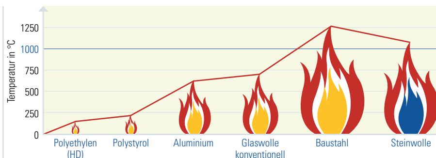
Schmelzpunkt von Baustoffen
