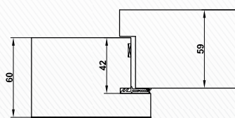
Exécution à recouvrement
