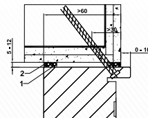
Cadre applique PL CombiModul
