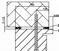
Cadre applique PM CombiModul
