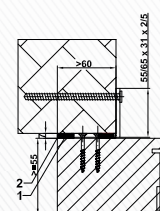
Cadre applique PM CM, équerre vissée
