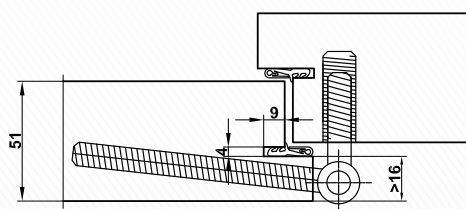
CompactPrestige (Alu) 51mm Compact WinTop 51mm AluTop Plus 51mm
