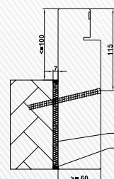
Cadre bloc PM en saillie
