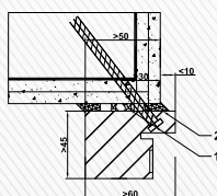
Cadre applique PL avec coupe transversale réduite
