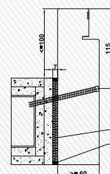
Cadre bloc PL en saillie
