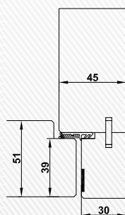
Cadre embrasure BLOTool BF
