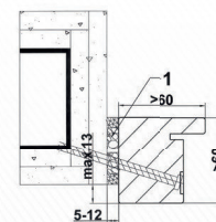
Cadre bloc PL CombiModul, cadre en sailli av. acryl coupe-feu / silicone
