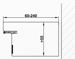
CombiModul cadre bloc avec élargissement cadre
