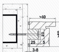
Cadre bloc PL CombiModul av. baguette montage bois massif av. acryl coupe-feu / silicone
