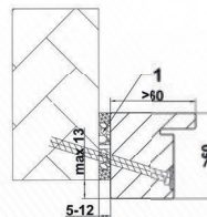
Cadre bloc PM CombiModul, cadre en sailli av. acryl coupe-feu / silicone
