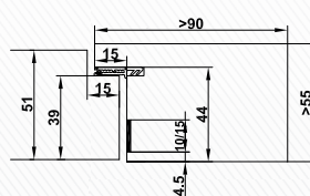
Cadre applique CombiModul
