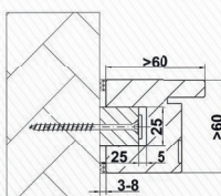
Cadre bloc PM CombiModul av. baguette montage bois massif av. acryl coupe-feu / silicone
