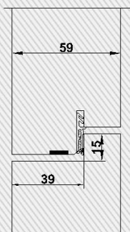
Vertikalschnitt Türblatt / Oberblende überfäلت
