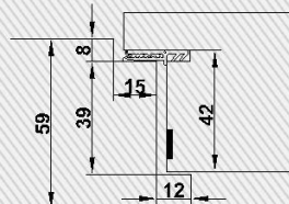
CombiModul überfäلت Horizontalschnitt Türblatt - Rahmen
