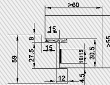
CombiModul-Blockrahmen Reduzierte Falztiefe 1-flg ohne Glas B_{\max} = 1050\text{mm} ; H_{\max} = 2200\text{mm}
