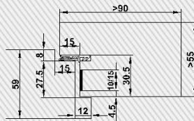
CombiModul-Blendrahmen Reduzierte Falztiefe 1-flg ohne Glas B_{\max} = 1050\text{mm} ; H_{\max} = 2200\text{mm}
