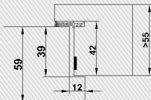
CombiModul überfäلت Horizontalschnitt Türblatt - Rahmen
