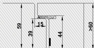
CombiModul stumpf Horizontalschnitt Türblatt - Rahmen
