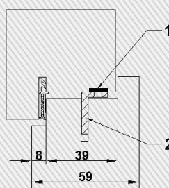
CombiModul überfäلت Vertikal- und Horizontalschnitt Oberblende - Rahmen
