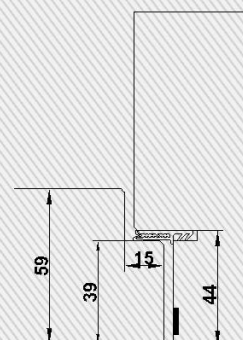
BLOCTool Horizontalschnitt Türblatt - Rahmen
