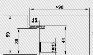
CombiModul-Blendrahmen
