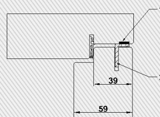
BLOCTool Vertikal- und Horizontalschnitt Oberblende - Rahmen
