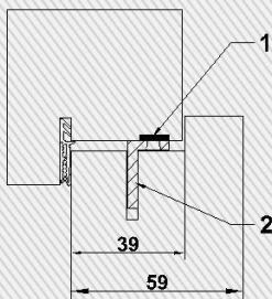
CombiModul überfäلت Vertikal- und Horizontalschnitt Oberblende - Rahmen
