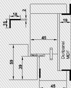
Blockfutter mit Futterbrett Alu-Winkel BLOTool BL
