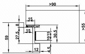
CombiModul-Cadre applique prof. battue réd. 1 vant. sans verre Larg. max =1050mm; Haut. max =2200mm
