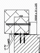
Cadre applique PM CM, équerre vissée
