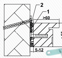
Cadre bloc PM CombiModul avec équerre Z
