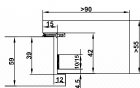
Cadre applique CombiModul
