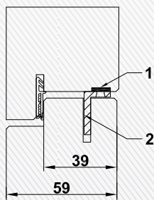
CombiModul affleuré Coupe verticale et horizontale Attique - Cadre
