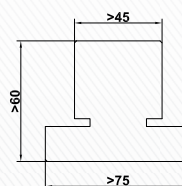
Meneau / Travers sans branchement
