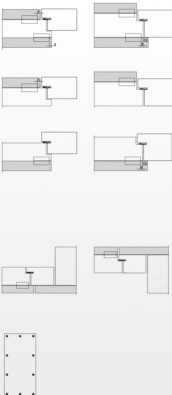
Arrangements des ferrages Doplex
