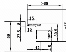
CombiModul-Cadre bloc prof. battue réd. 1 vant. sans verre Larg. max =1050mm; Haut. max =2200mm
