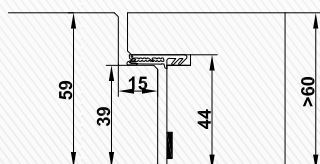
CombiModul affleuré Coupe horizontale Panneau porte - cadre
