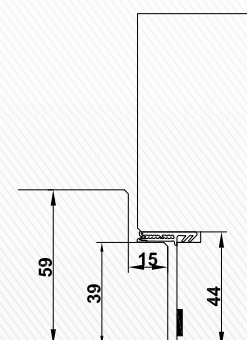
BLOCTool Coupe horizontale Panneau porte - cadre
