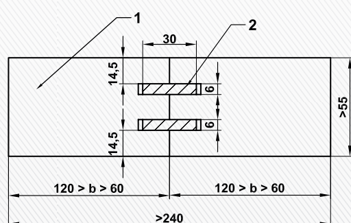
CombiModul cadre applique avec élargissement cadre
