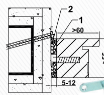
Cadre bloc PL CombiModul avec équerre Z
