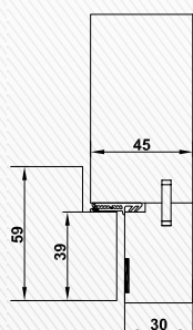
Cadre embrasure BLOTool BF
