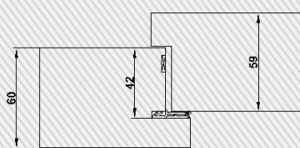
Ausführung mit Überschlag
