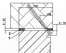
Blendrahmen MBW CombiModul
