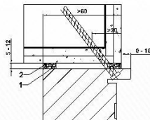
Blendrahmen LBW CombiModul
