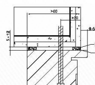
Blendrahmen LBW CombiModul
