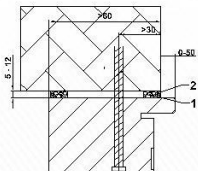
Blendrahmen MBW CombiModul
