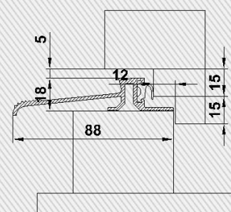
Typ H4, mit HEBGO 160/620 (mit Schwellenholz Eiche)
