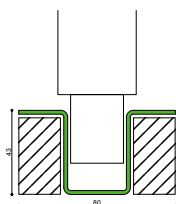
RAIL INFÉRIEUR DE TYPE ENCASTREMENT
