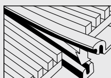
STEWELL CLIPFIX zur längseitigen Verbindung von Mattenbahnen
