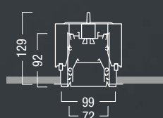
MRT Einbaukanal mit umlaufendem Rahmen
