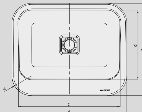
Variante de montage A* (bord large = côté face à l'utilisateur)
