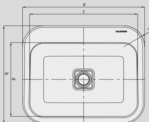
Variante de montage B* (bord étroit = côté face à l'utilisateur)
