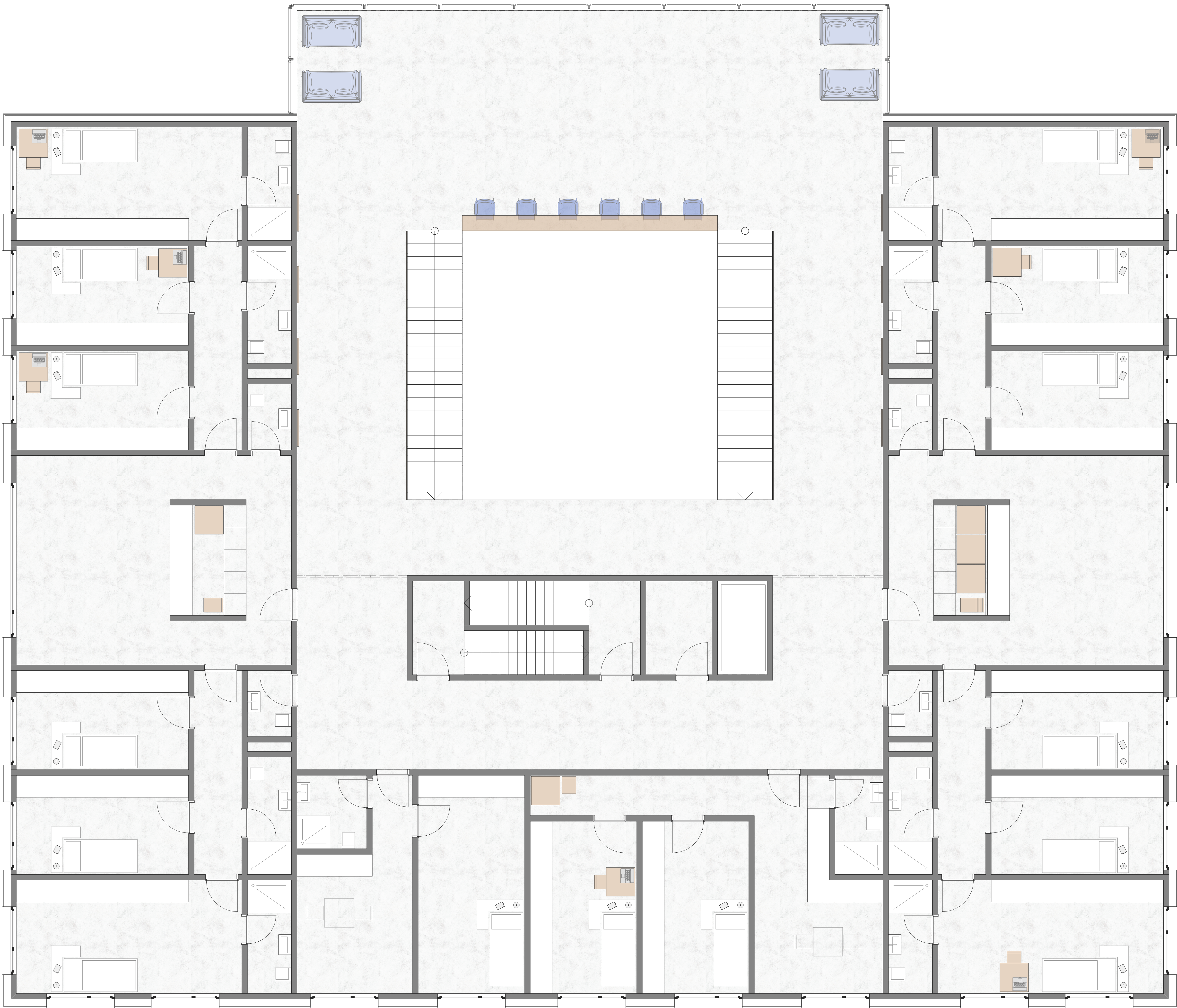
Grundriss 3. Obergeschoss 1:50
