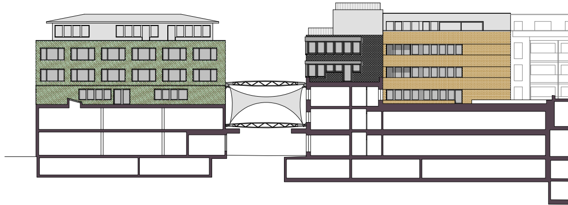
Querschnitt
