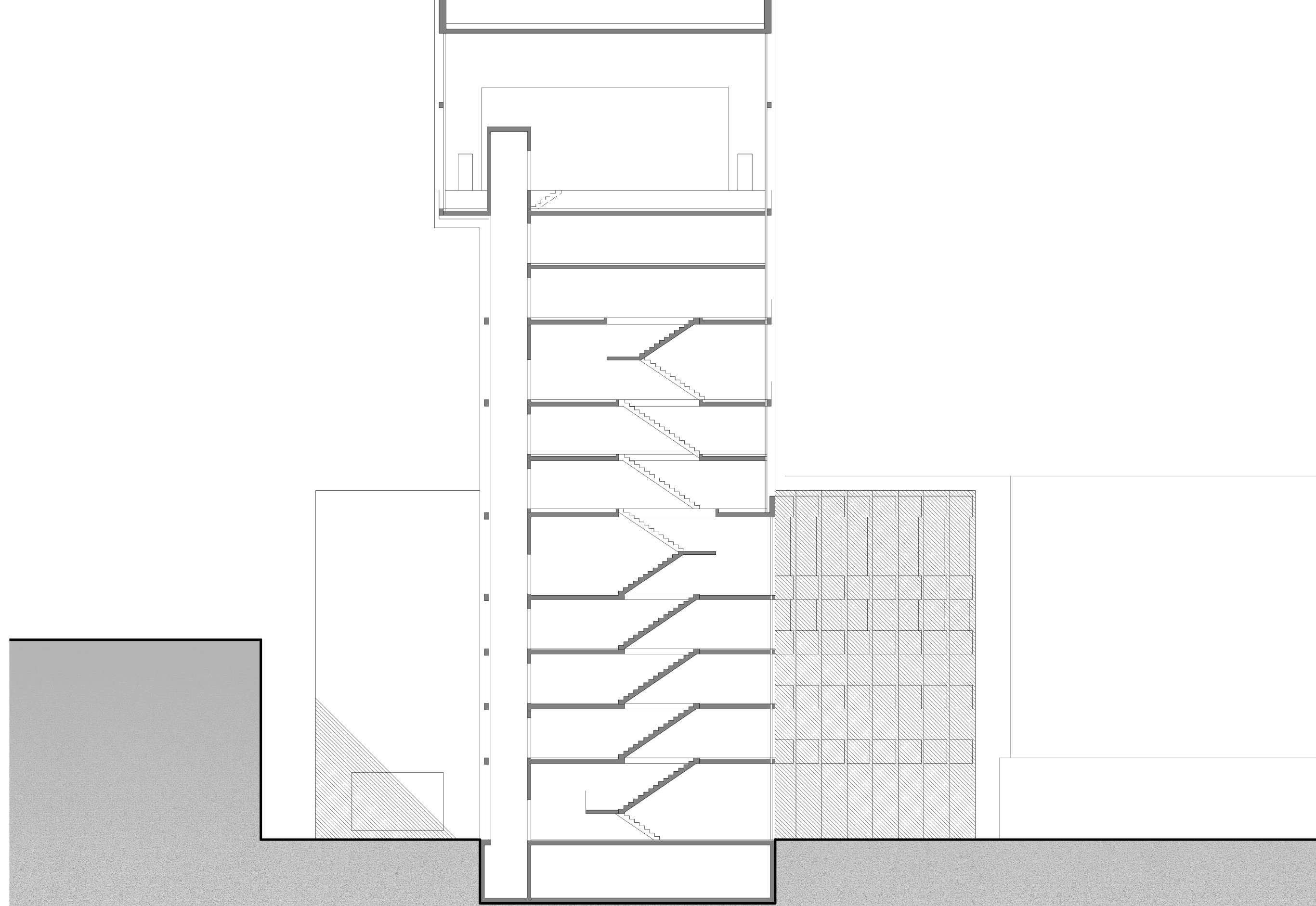
Querschnitt D-D Treppen Kern 1:200
