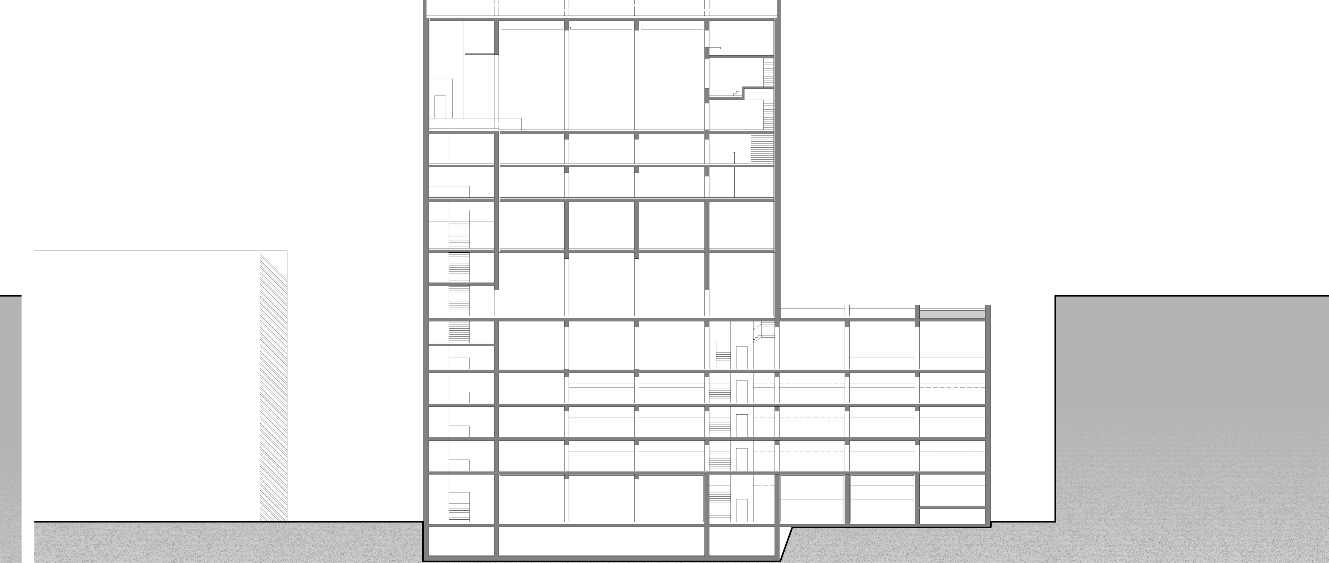
Querschnitt A-A 1:200
