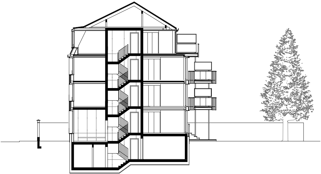
Querschnitt
