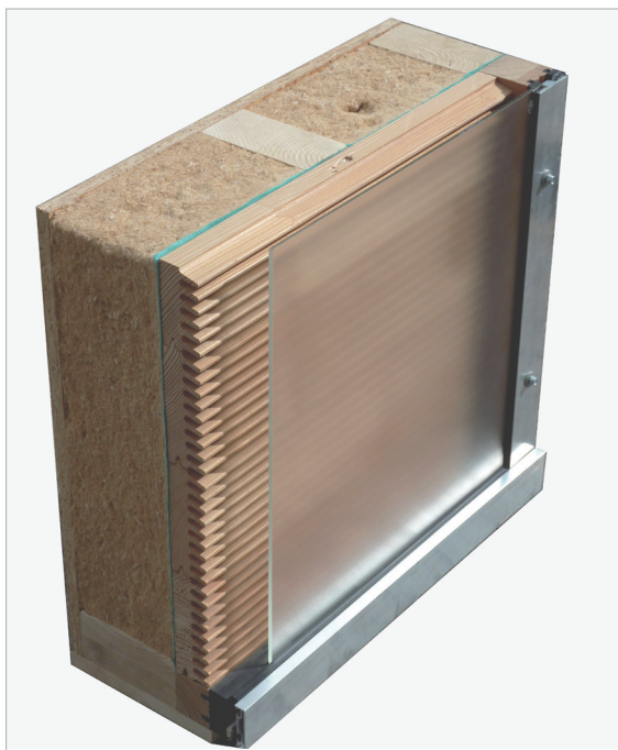
détail structurel
