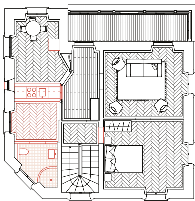
2ème étage 1:200
