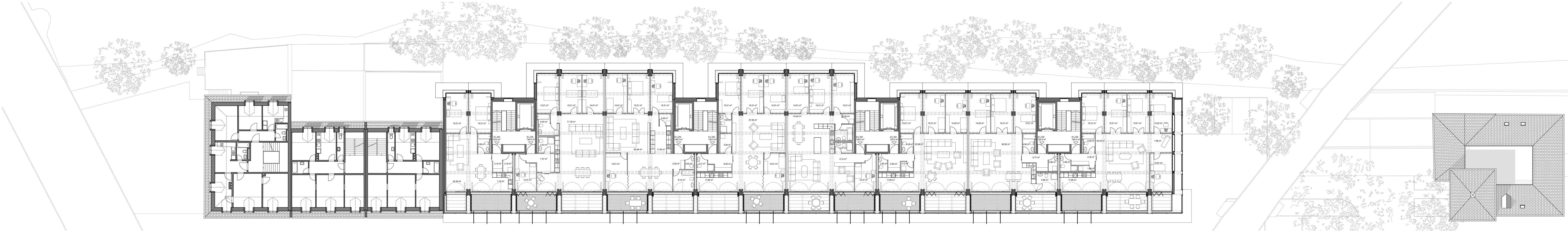
Grundrissplan OG_Variante Wohnungen 1:200
