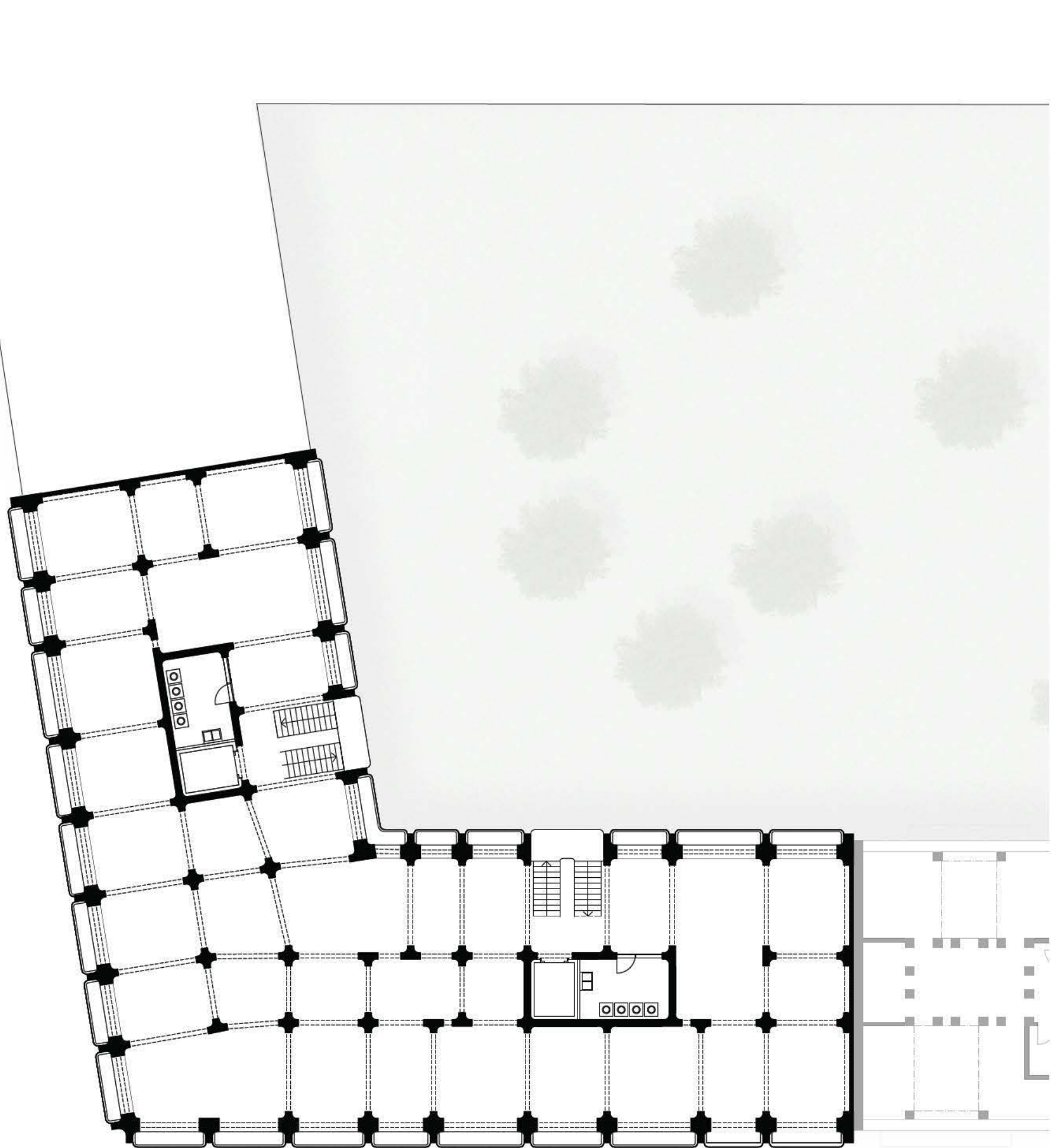
Grundriss Dachgarten 1.200
