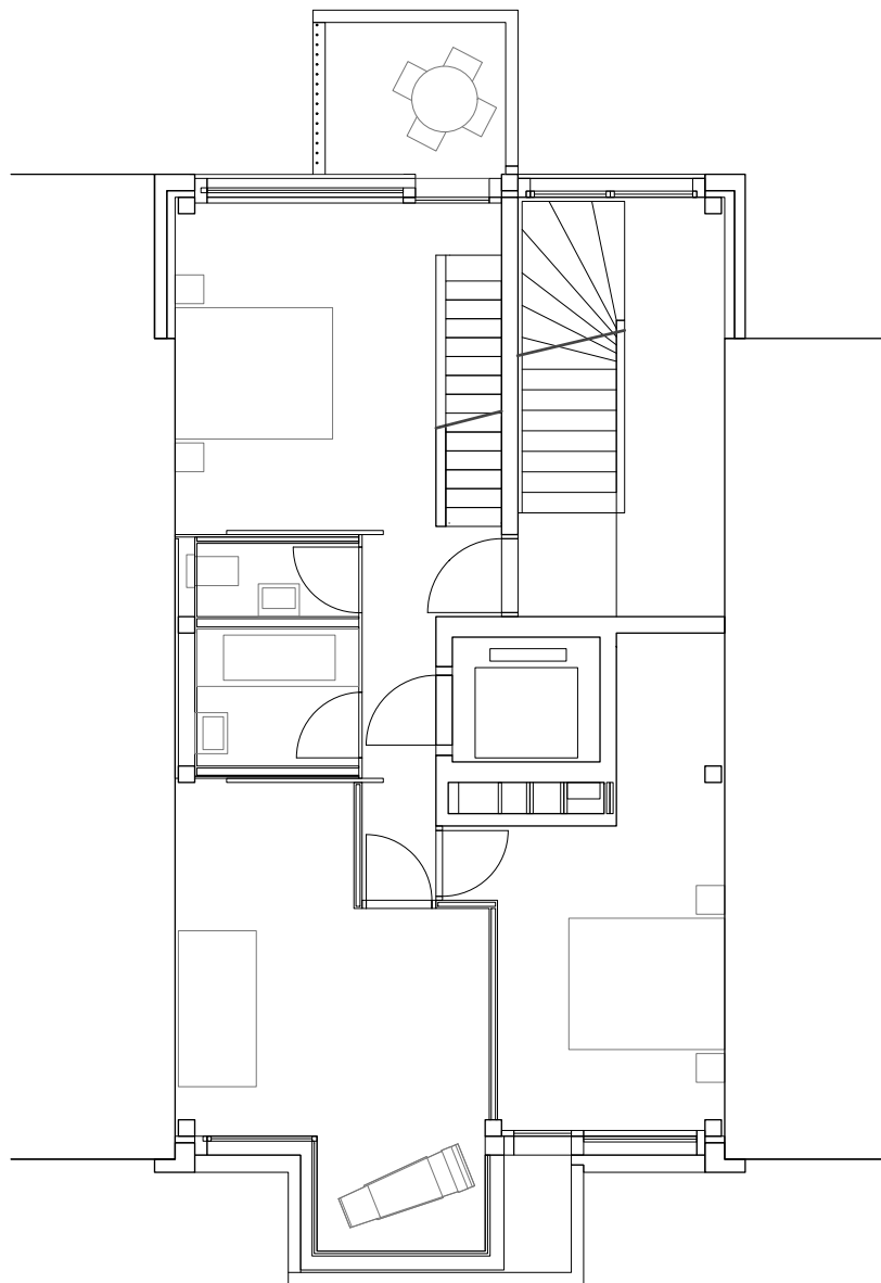
1. Obergeschoss 1:100
