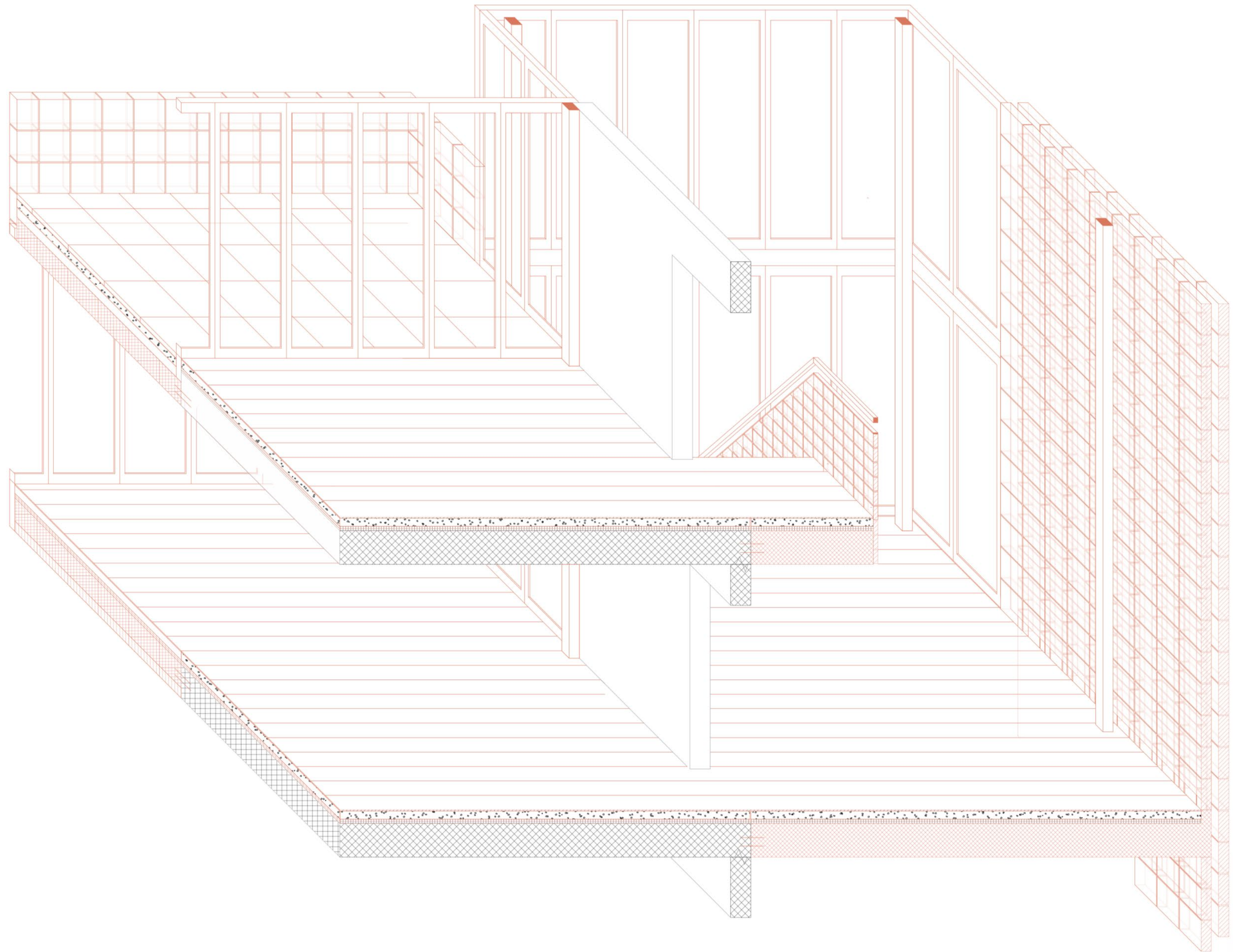
Detailschnitt Anbau 1:20
