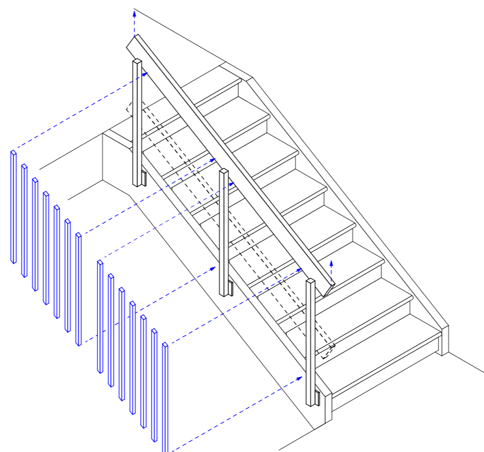
Umbau bestehendes Geländer 1. Oberster Handlauf auf 90cm erhöhen 2. Unteren Handlauf entfernen 3. Flächen mit übrigen Holzleisten füllen
