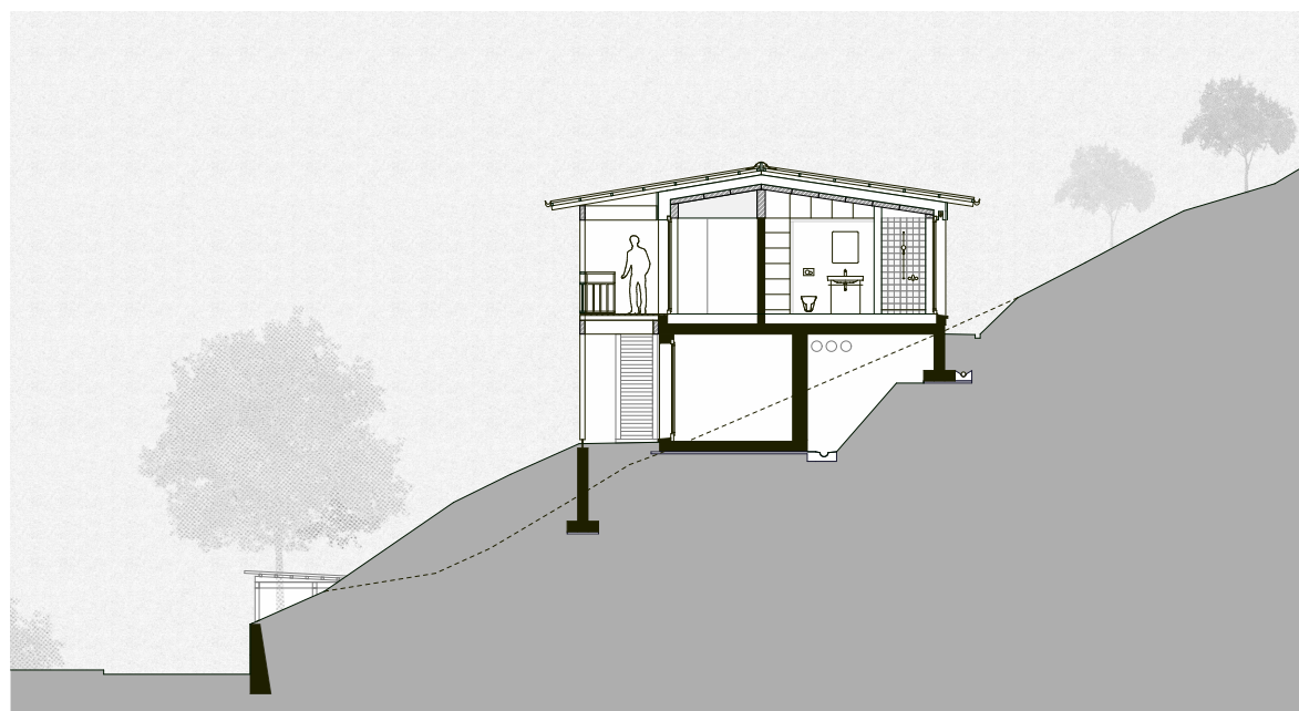
Längs-und Querschnitt 1:200
