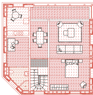
Surélévation 1:200
