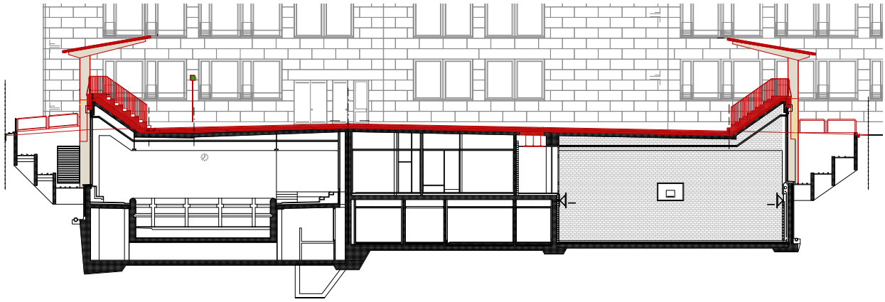
Längsschnitt durch das Untergeschoss , Mst. 1:450, links die Schwimm-, rechts die Turnhalle. Gut erkennbar sind die typisch abgeknickten Unterzüge im Fassadenbereich. Die jeweils sechs neuen Betonstützen, die die Tribünendächer tragen, sind nahtlos an die bestehende Tragkonstruktion angefügt und mit Schrauben in den innen liegenden Betonträgern rückverankert.
