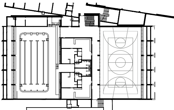
Sporthalle, Grundriss UG , Mst: 1:800. Links liegt die Schwimm-, rechts die Turnhalle. Dazwischen befinden sich die Garderoben, die an die Schulhäuser Vogesen (oben) und St. Johann (unten) anschliessen.
