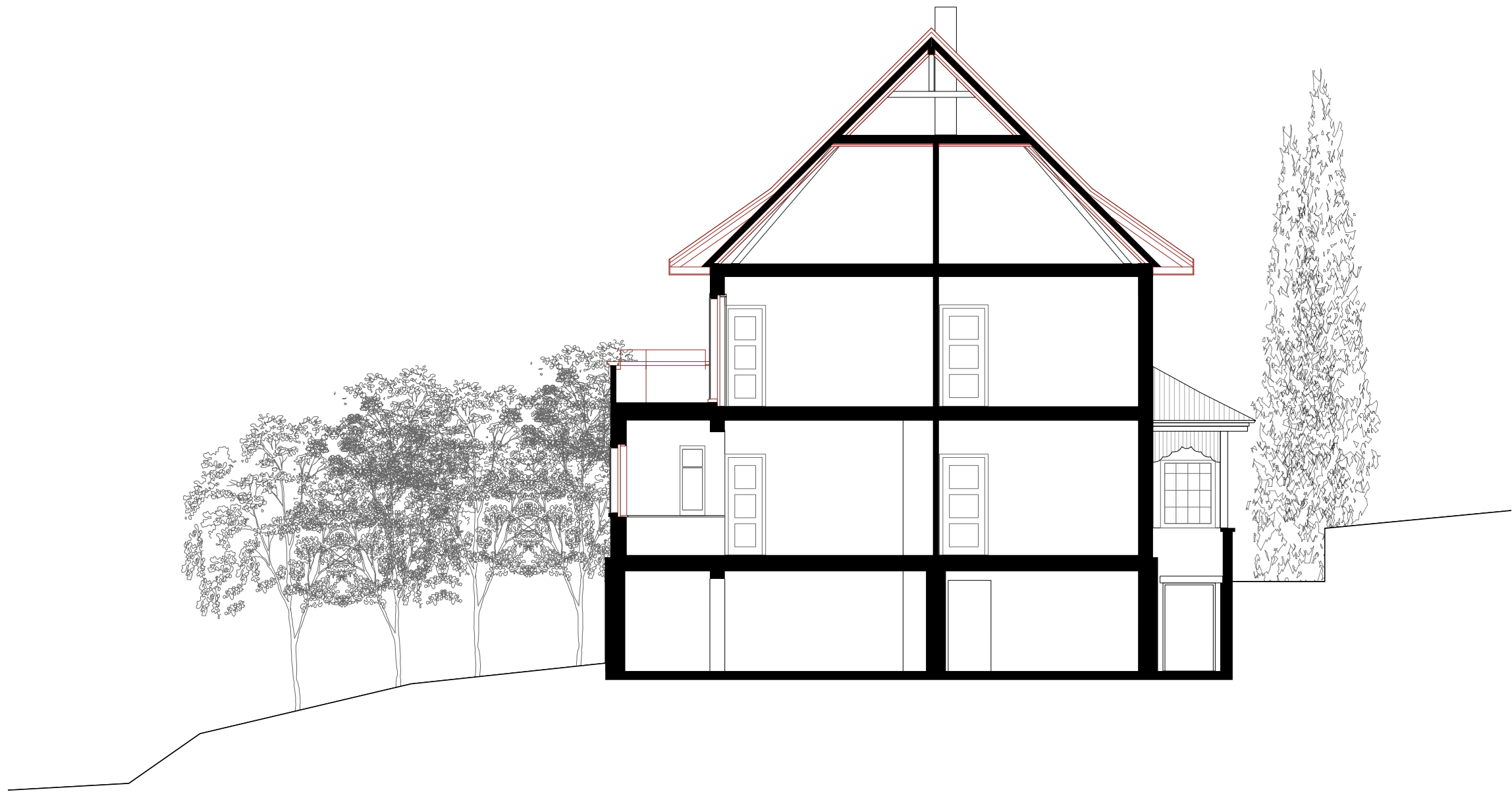
Schnitt 1:100
