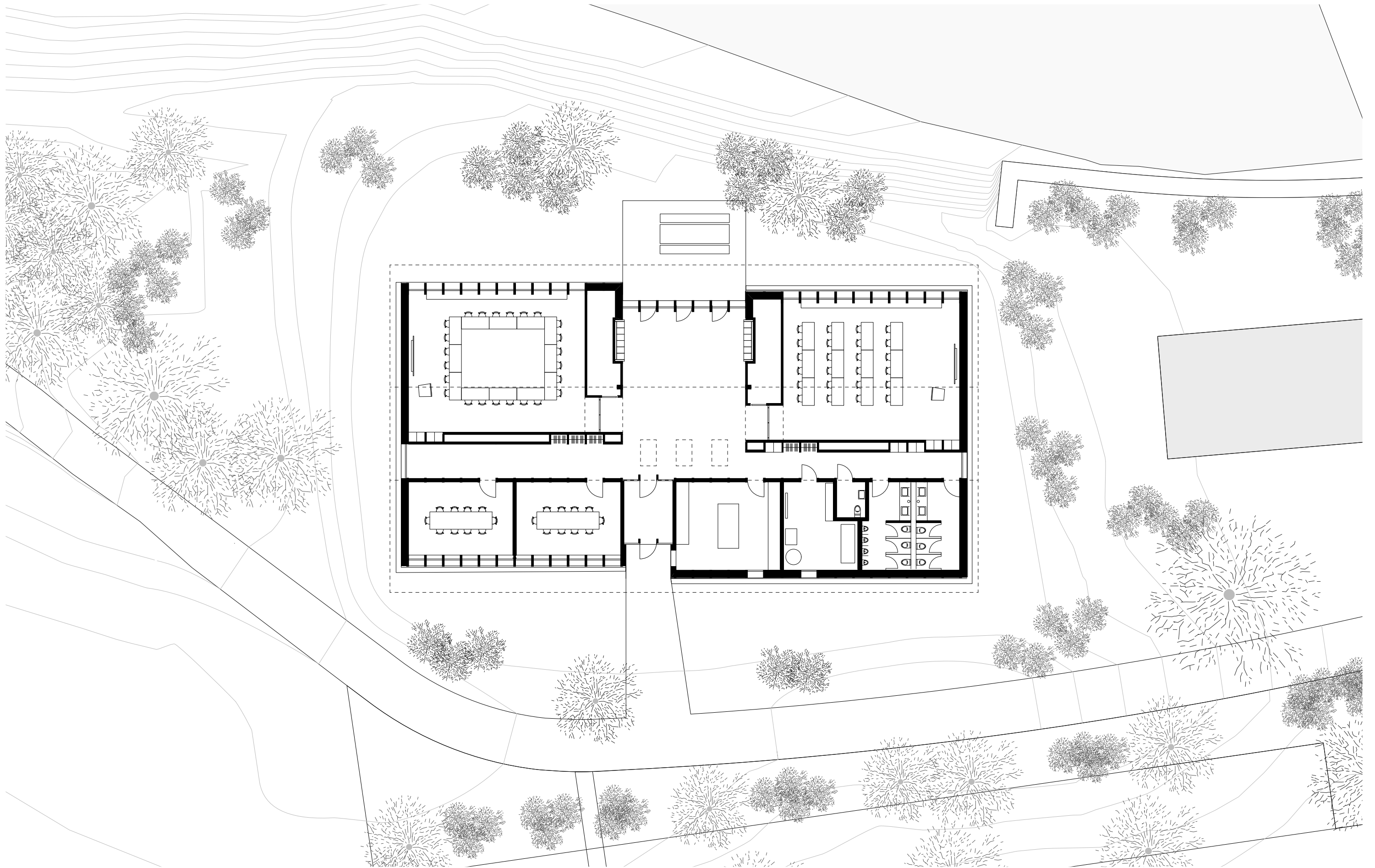
Grundriss Erdgeschoss
