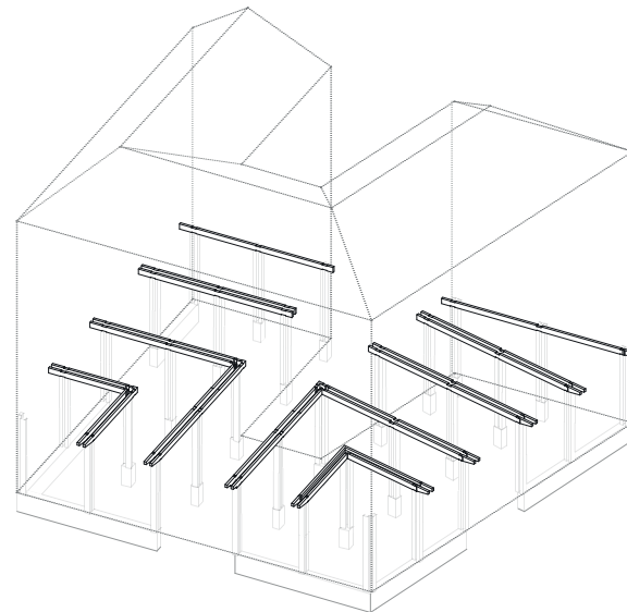
2. Primärträgerpaare
