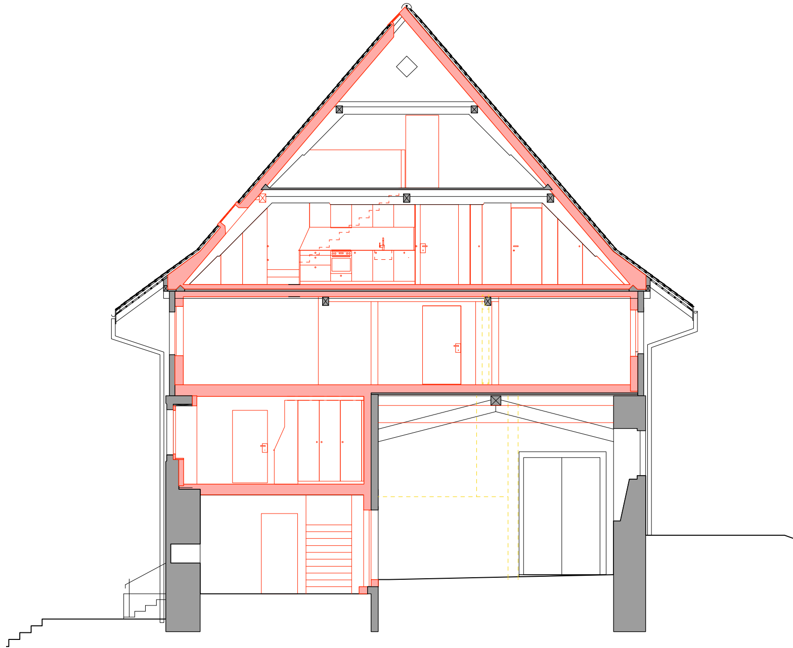
Querschnitt AA 1:100
