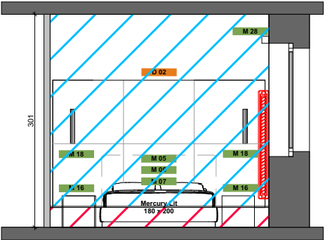
ELEVATION A-A1
