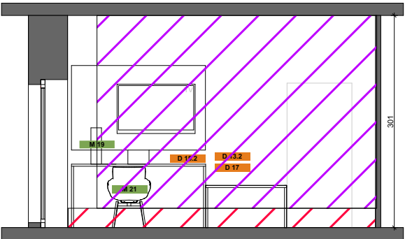
ELEVATION B-B
