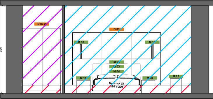
ELEVATION A-A
