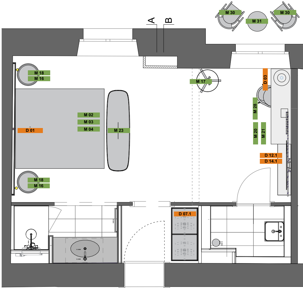
PLAN CHAMBRE 1:50
