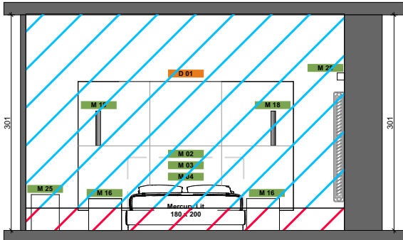
ELEVATION A1-A1 1: 75
