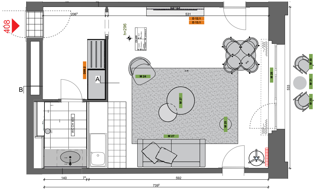
PLAN CHAMBRE 1:50 REPERAGE SUR PLAN CHAMBRE N° 408 Surface: 44m²
