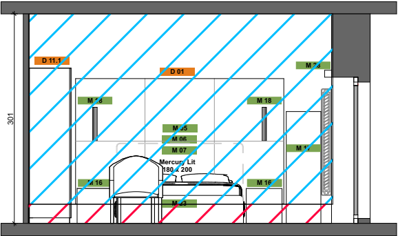
ELEVATION A-A
