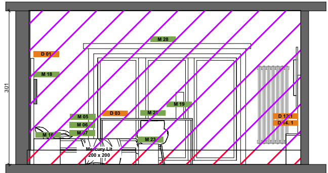
ELEVATION C-C
