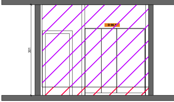
ELEVATION D-D
