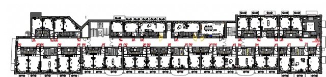
PLATEAU 3/ ETAGE 3
