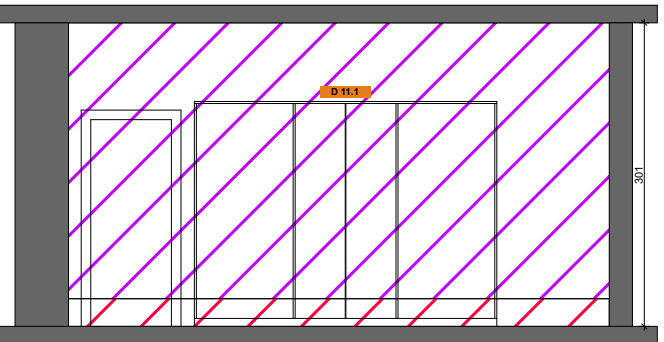
ELEVATION C-C
