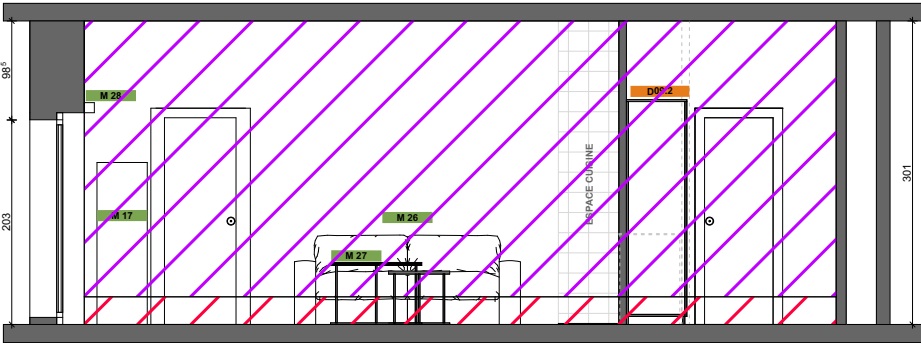
ELEVATION B-B 1:75
