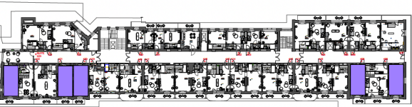
PLATEAU 3/ ETAGE 4
