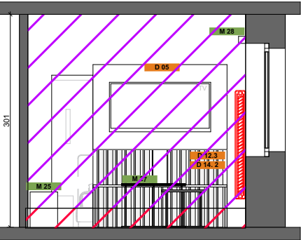
ELEVATION A-A
