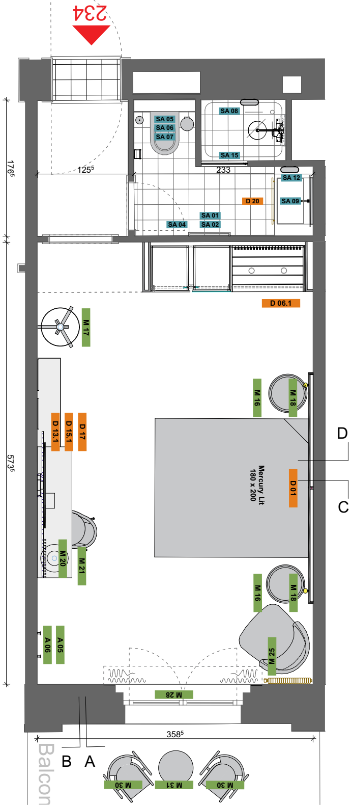
PLAN 1:50
