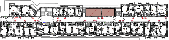
PLATEAU 3/ ETAGE 4
