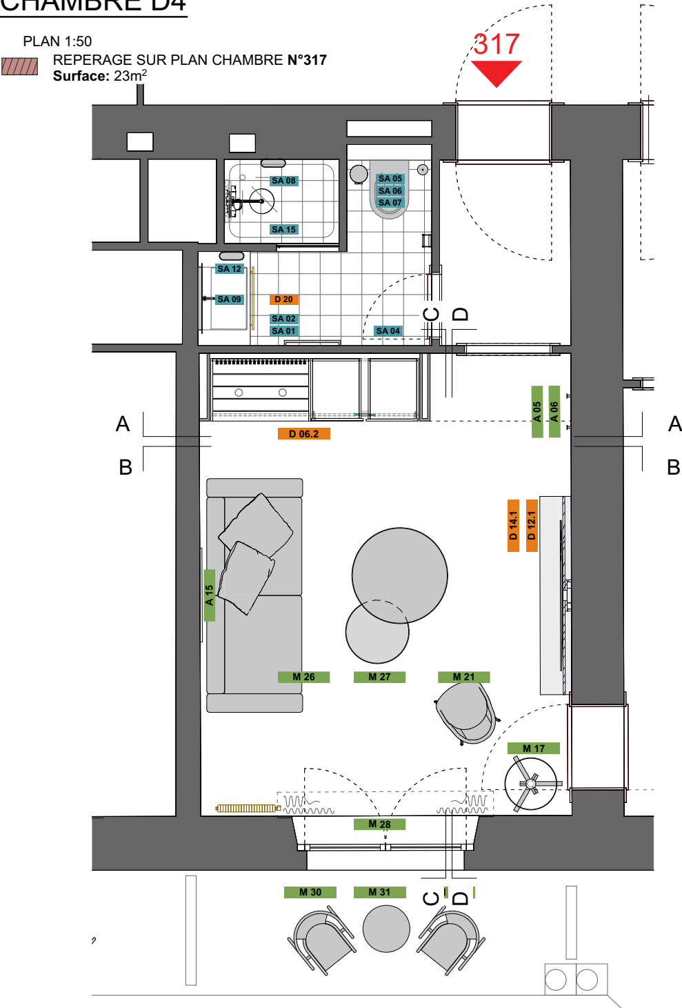
PLATEAU 3/ ETAGE 1
