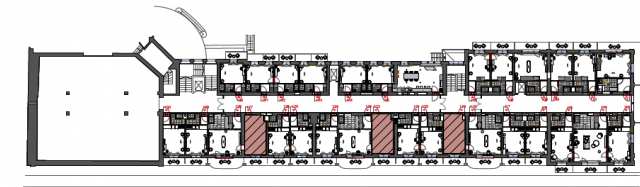
PLATEAU 3/ ETAGE 3
