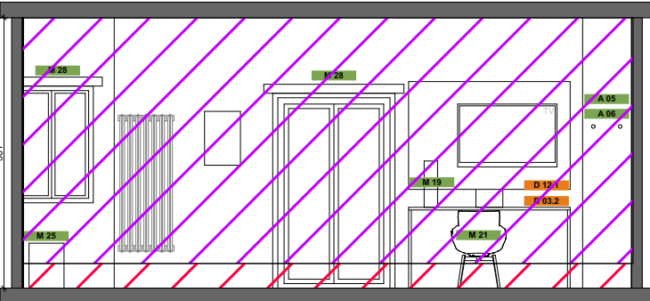
ELEVATION C-C
