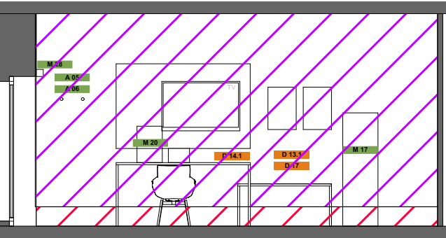
ELEVATION B-B
