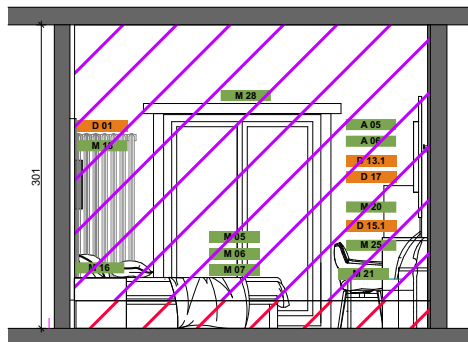
ELEVATION C-C
